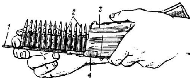
Рис. 56. Снаряжение магазина патронами из обоймы: 1 — обойма; 2 — патроны; 3 — магазин; 4 — переходник
