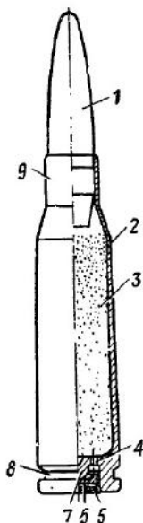
Рис. 36. Боевой патрон:
