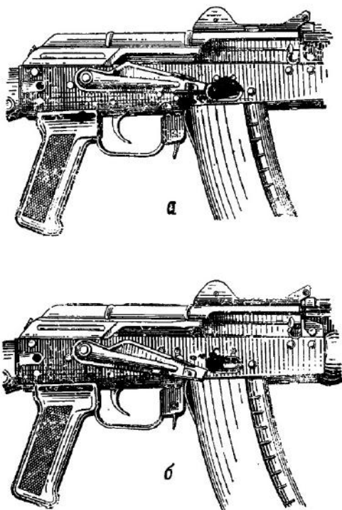
Рис. 60. Установка переводчика на необходимый вид огня:
