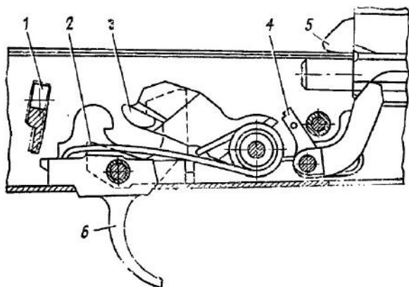
Рис. 38. Положение частей ударно-спускового механизма до заряжания при включенном предохранителе и спущенном курке:
