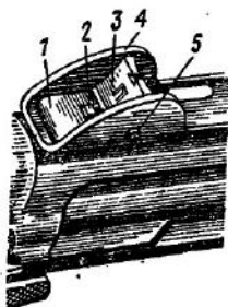
Рис. 25. Поворотный целик:
