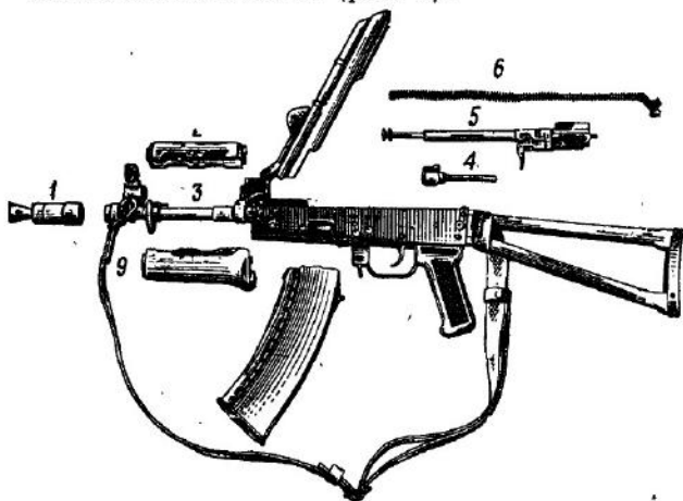
Рис. 2. Основные части и механизмы автомата:
