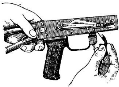
Рис. 16. Извлечение автоспуска с пружиной из ствольной коробки
