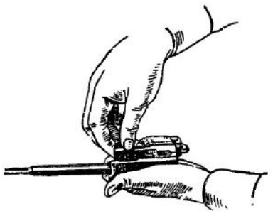
Рис. 8. Отделение затвора от затворной рамы
