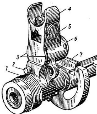
Рис. 23. Основание мушки:
