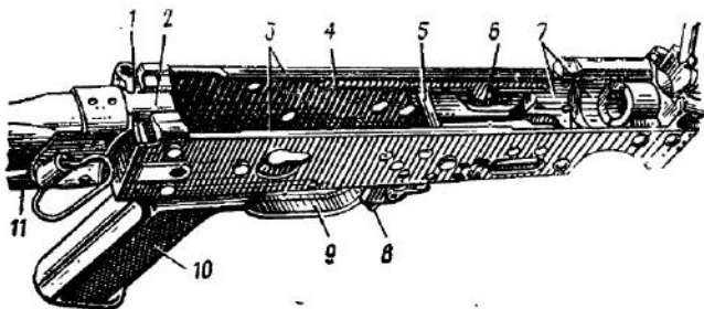
Рис. 24. Ствольная коробка:
