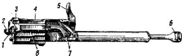
Рис. 28. Затворная рама с газовым поршнем:
