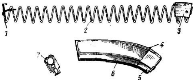
Рис. 34. Магазин:
