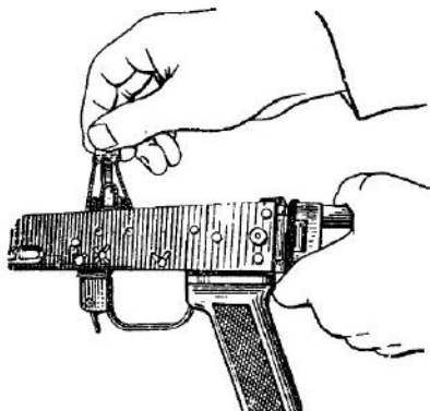
Рис. 15. Извлечение курка из ствольной коробки
