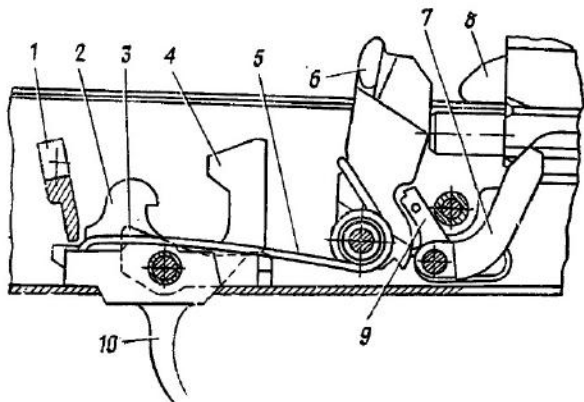
Рис. 39. Положение частей ударно-спускового механизма перед выстрелом:
