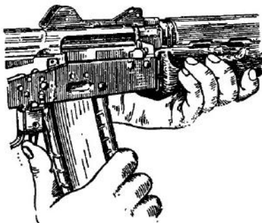
Рис. 3. Отделение магазина
