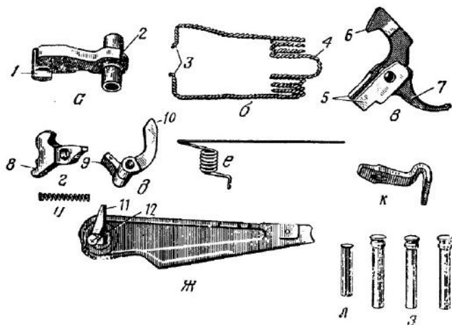
Рис. 32. Части ударно-спускового механизма:
