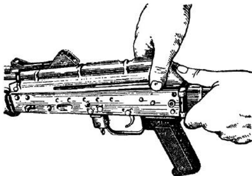
Рис. 5. Открывание крышки ствольной коробки
