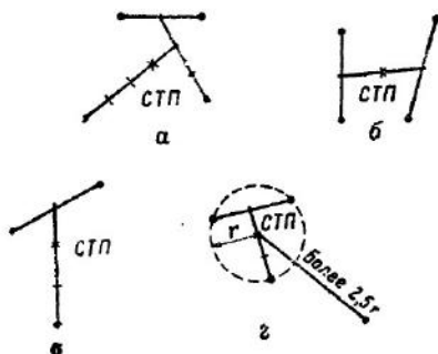
Рис. 45. Определение средней точки попадания:
