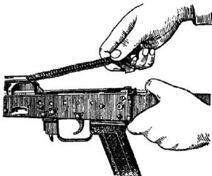
Рис. 6. Отделение возвратного механизма
