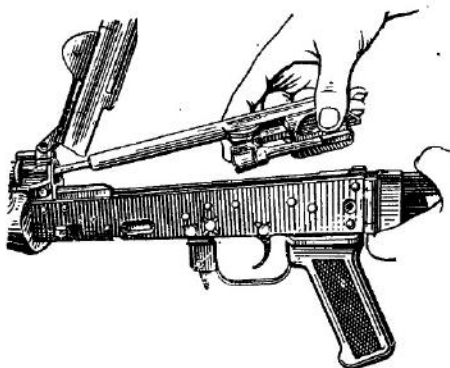
Рис. 7. Отделение затворной рамы с затвором
