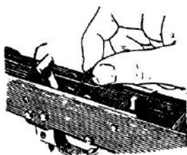
Рис. 13. Заведение правого конца боевой пружины за боевой взвод курка
