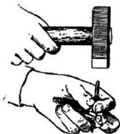
Рис. 12. Выталкивание шпильки при отделении выбрасывателя и ударника от затвора
