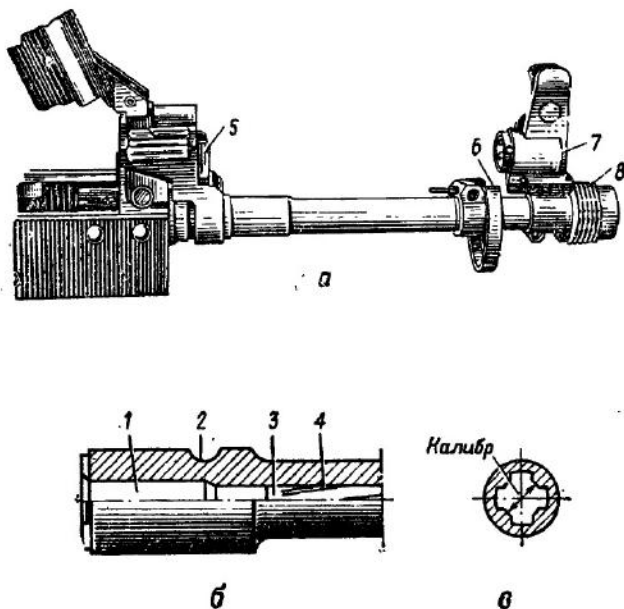
Рис. 21. Ствол:
