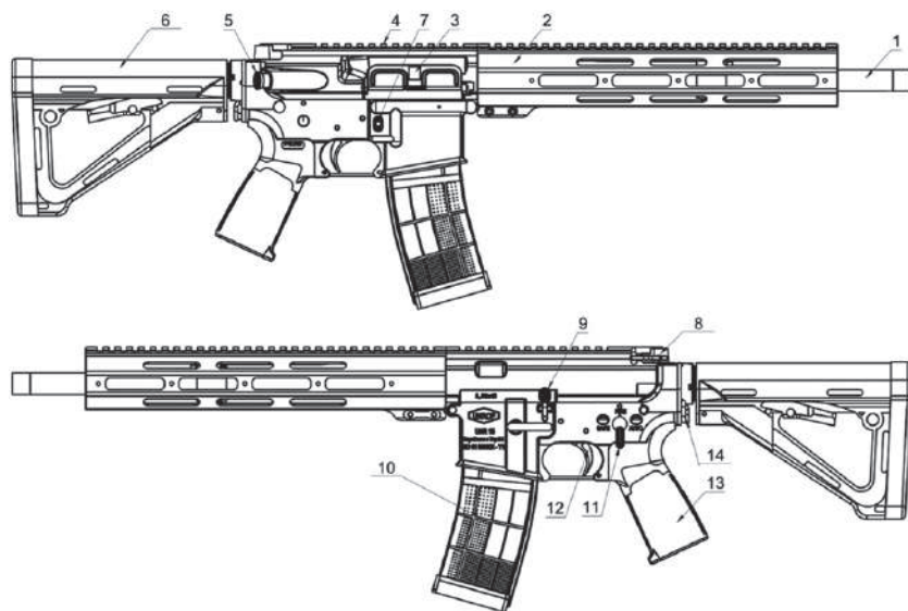
Рис. 70. Органи керування та елементи будови
