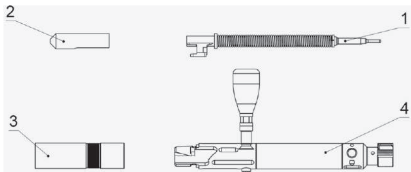
Рис. 141. Затвор у розібраному стані:
