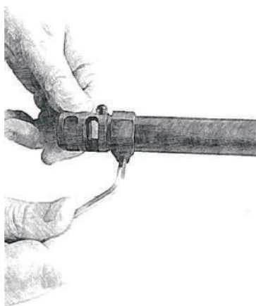
Рис. 41. Фіксація дульного гальма-компенсатора
