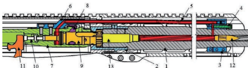
Рис. 9. Схема принципу роботи автоматики
