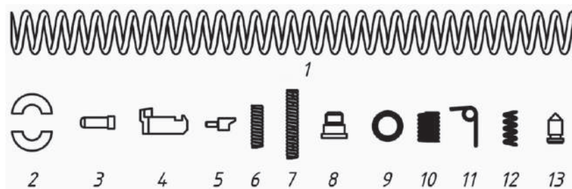
Рис. 175. Комплект деталей для ремонту та заміни деталей
