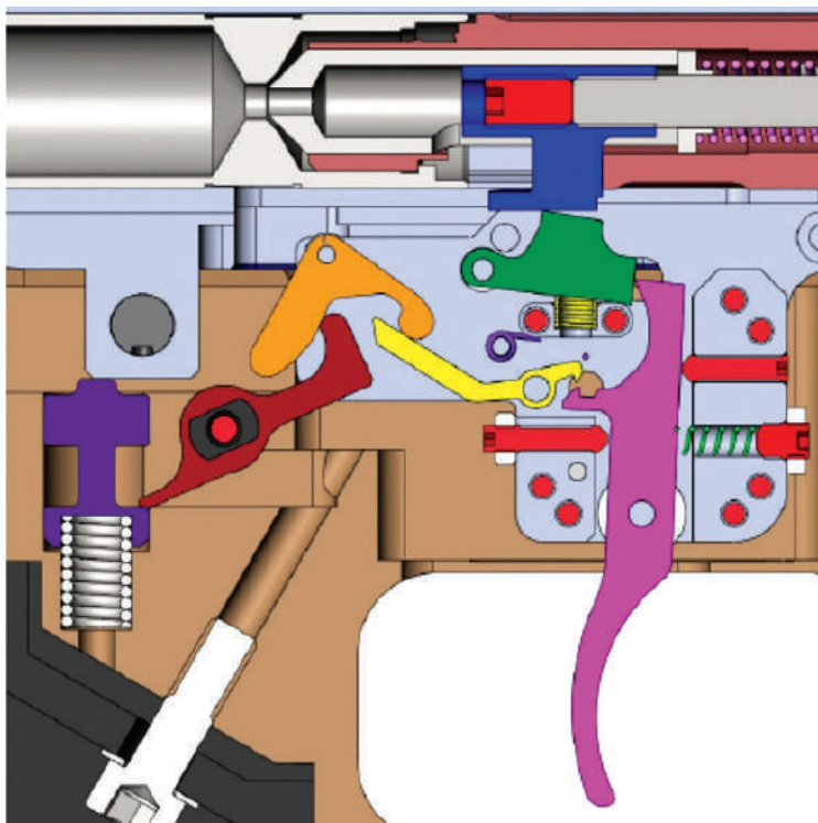
Рис. 149. Положення деталей ударно-спускового механізму і затвора після пострілу
