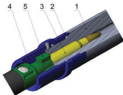
Рис. 147. Ствол із патронником та муфтою бойових упорів.
