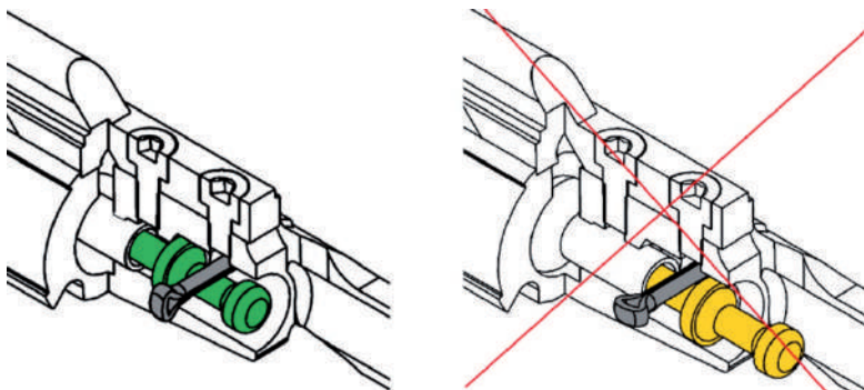
Рис. 94. Фіксація ударника шплінт під час збирання затворної рами
