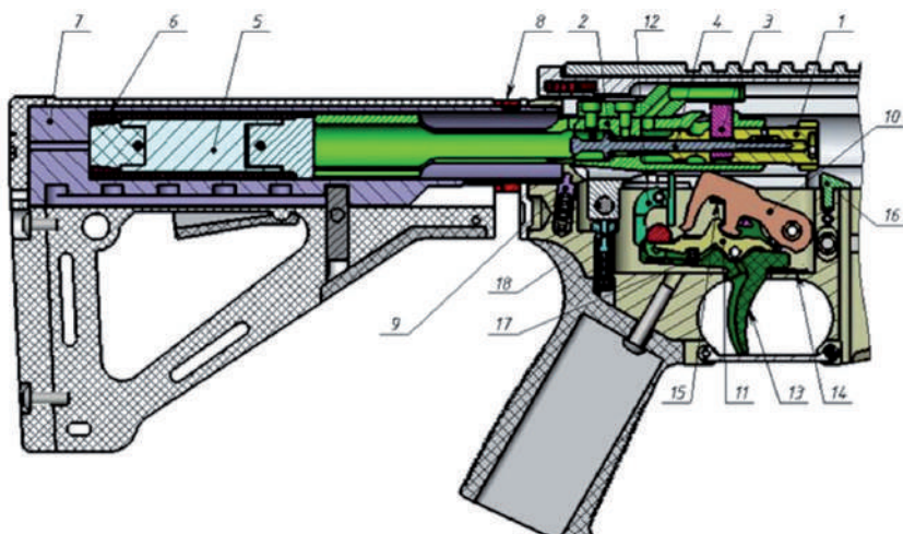
Рис. 75. Схема роботи автоматики UAR-15
