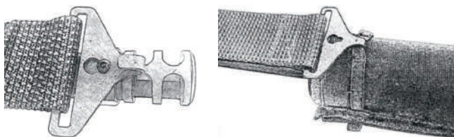
Рис. 55. Кріплення пряжки антиміражної стрічки: а) за дульне гальмо-компенсатор; б) за чохол глушника
