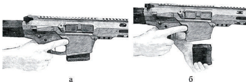
Рис. 11. Від'єднання магазину
