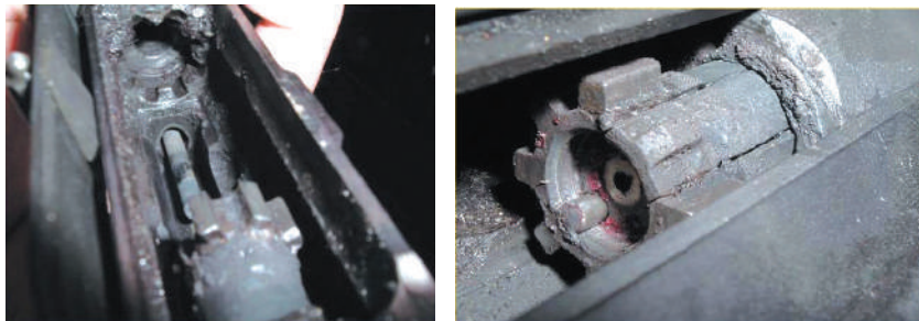
Рис. 125. Сильне забруднення голівки затвора та патронника
