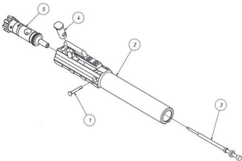
Рис. 18. Затворна рама у розібраному вигляді:
