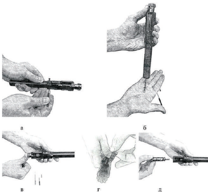
Рис. 17. Від'єднання затвора від затворної рами
