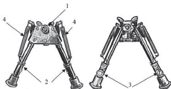
Рис. 44. Сошки:
