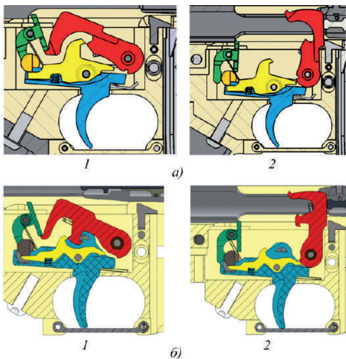
Рис. 104. Положення частин ударно-спускового механізму при натиснутому спусковому гачку в режимі автоматичної стрільби:
