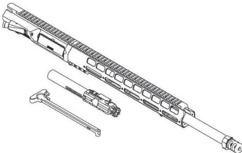
Рис. 16. Верхня рама ствольної коробки, затворна рама із затвором у зборі та важіль перезарядження
