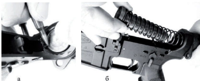
Рис. 87. Від'єднання буфера віддачі та зворотної пружини
