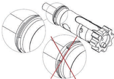
Рис. 23. Положення кілець на затворі
