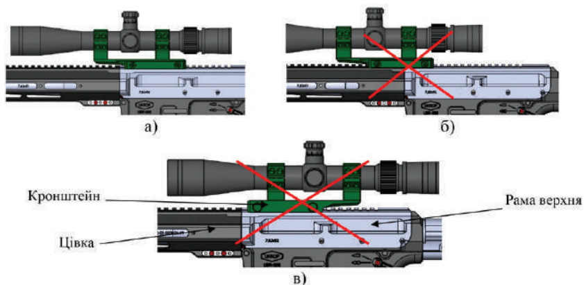
Рис. 162. Встановлення кронштейна на гвинтівку:
