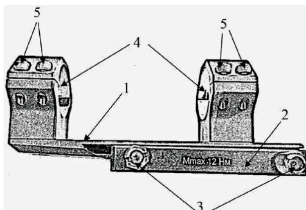
Рис. 161. Кронштейн для кріплення оптичного прицілу:
