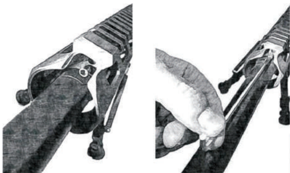
Рис. 62. Гвинт регулювання тиску порохових газів
