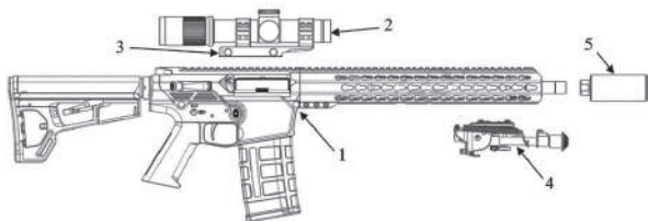
Рис. 4а. Гвинтівка UAR-10М з аксесуарами:
