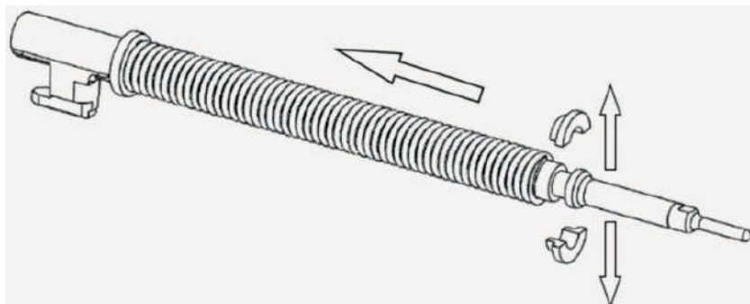
Рис. 152. Заміна пружини бойової:
