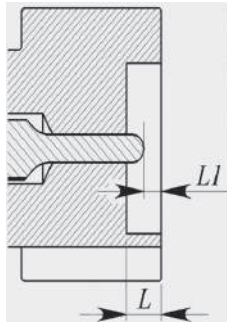
Рис. 171. Вихід бойка над дзеркалом затвора.
