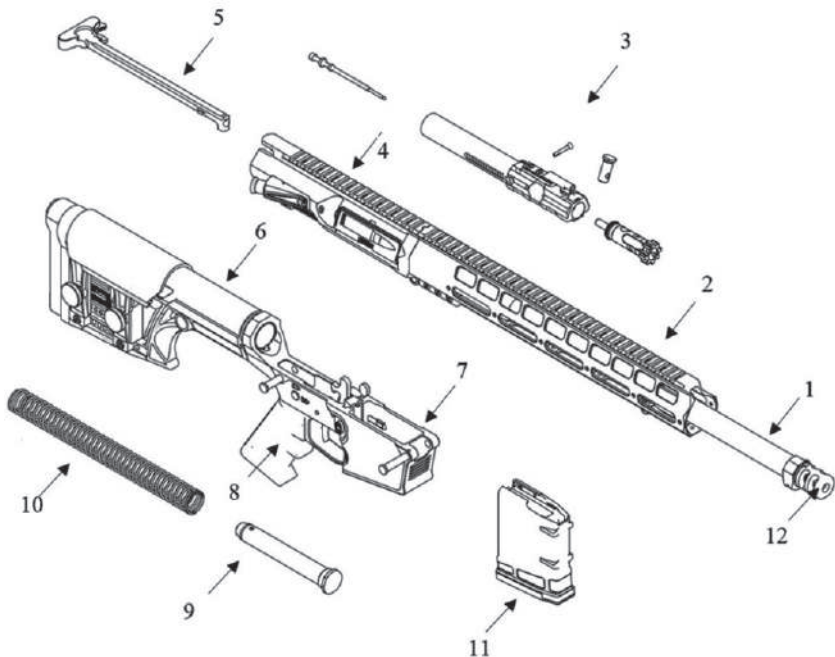
Рис. 21. Гвинтівка UAR-10 – неповне розбирання:
