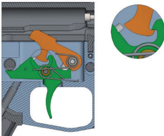
Рис. 33. Постановка курка на бойовий звід
