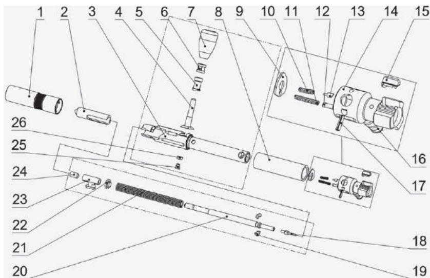
Рис. 153. Затвор (повне розбирання).
