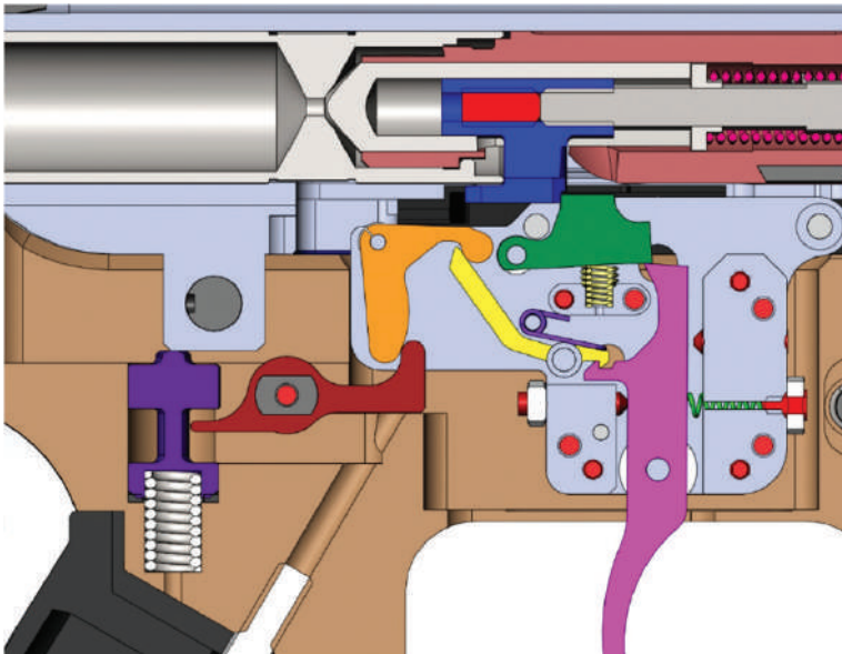
Рис. 151. Положення деталей ударно-спускового механізму при постановці на запобіжник
