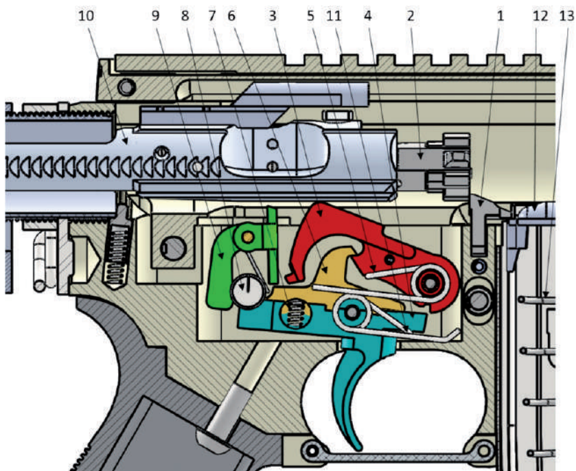
Рис. 107. Постановка затвора на затворну затримку:
