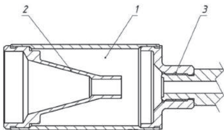
Рис. 112. Будова полум'ягасника:
