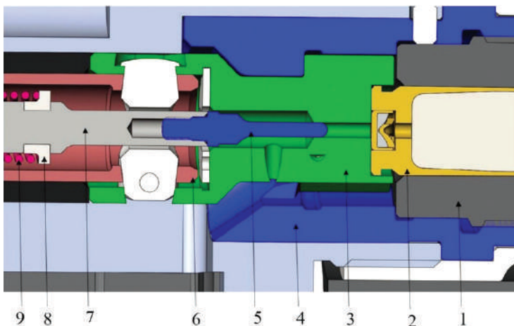
Рис. 146. Положення деталей затвора після заряджання:
