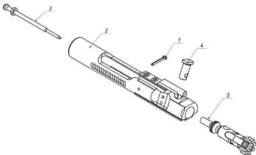
Рис. 86. Затворна рама у розібраному вигляді:
