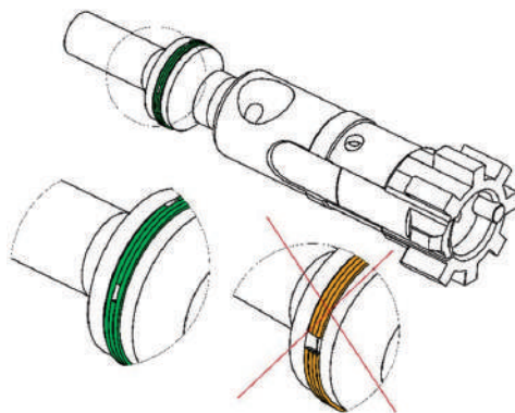
Рис. 93. Положення компресійних кілець на затворі
