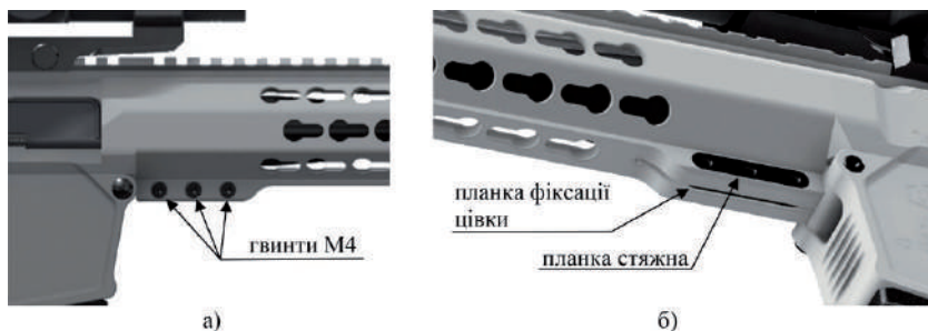
Рис. 63. Від'єднання цівки гвинтівки
