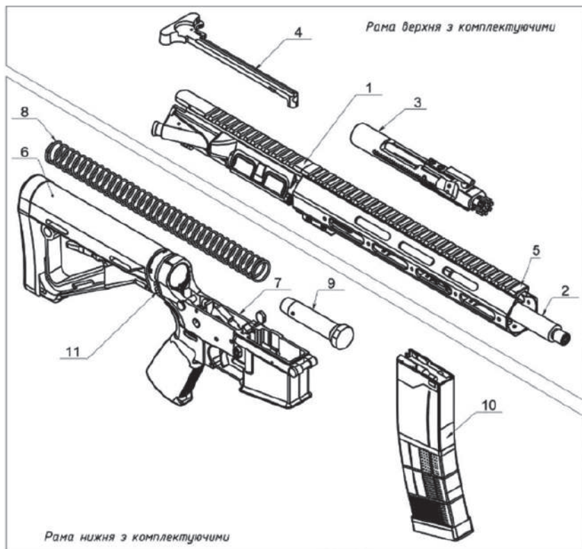
Рис. 71. Основні частини:
