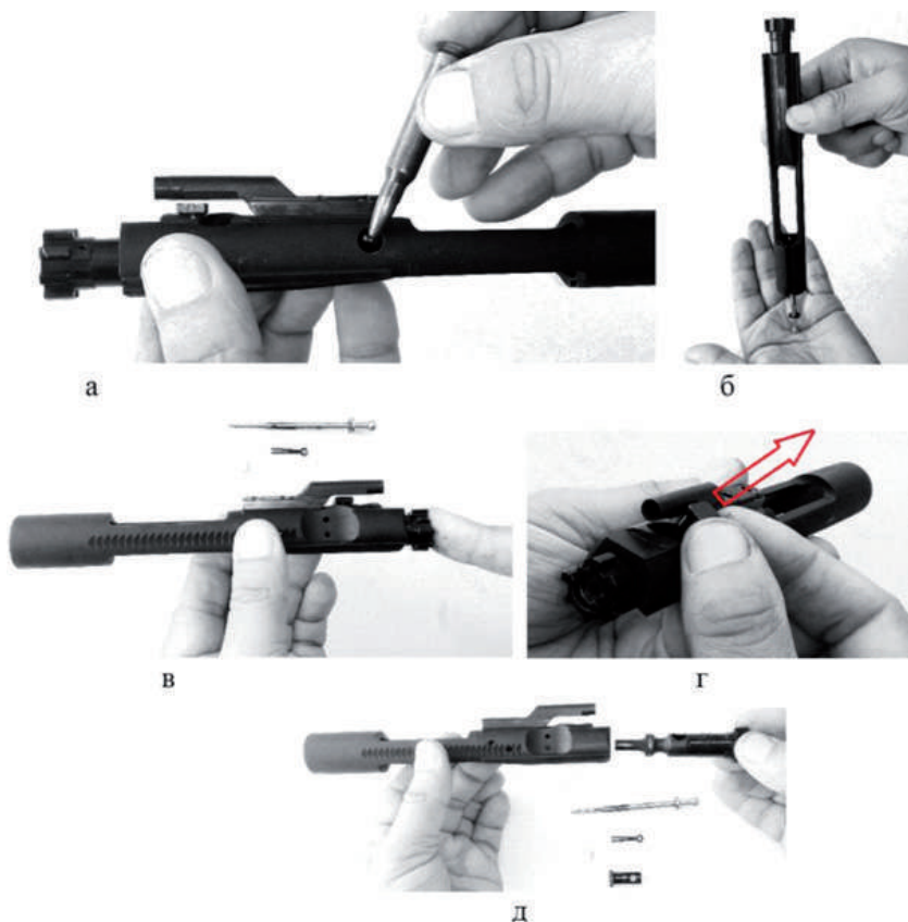
Рис. 85. Від'єднання затвора від затворної рами
