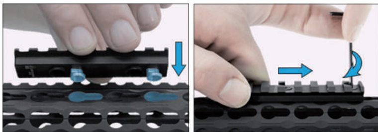
Рис. 6. Планка KeyMod, для кріплення додаткового обладнання
