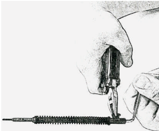
Рис. 172. Регулювання гвинта М6 та ударника
