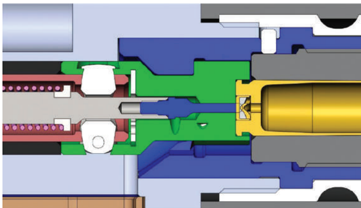
Рис. 150. Положення деталей затвора після пострілу
