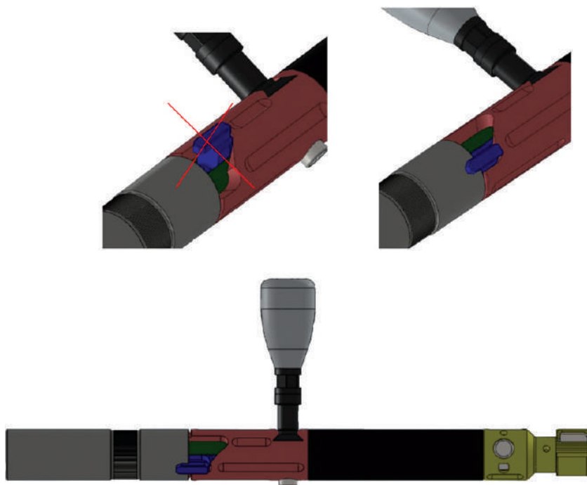
Рис. 143. Затвор у зібраному стані
