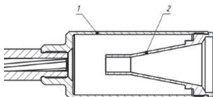
Рис. 43. Полум'ягасник:
