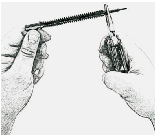
Рис. 173. Налаштування розміру виходу бойка
