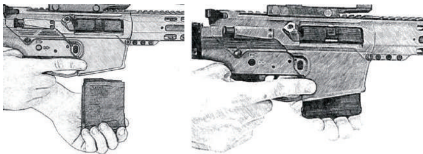
Рис. 26. Приєднання магазину до гвинтівки
