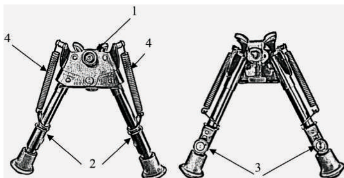
Рис. 158. Сошки:
