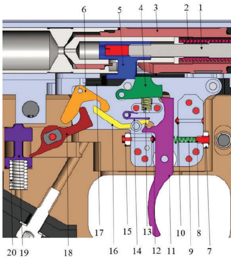
Рис. 148. Положення деталей спускового механізму і затвора після заряджання:
