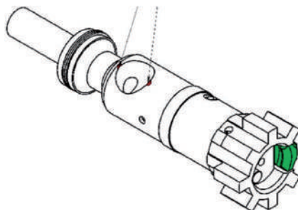
Рис. 92. Місце виступів на затворі, для запобігання неправильного збирання затворної групи
