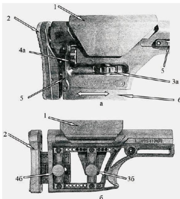
Рис. 164. Приклад та його основні частини: а) – Magpul PRS AR10/SR25; б) – Luth-AR MBA-1;
