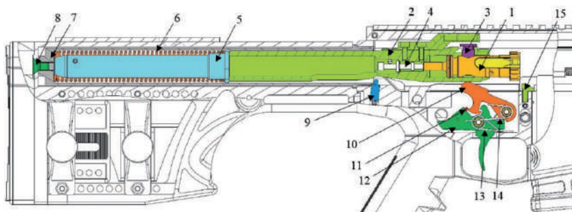
Рис. 10. Схема принципу роботи автоматики на прикладі UAR-10 (положення затвор розчеплений з муфтою бойових упорів, затворна рама знаходиться в задньому положенні, зворотна пружина стиснута, спусковий гачок натиснутий)
