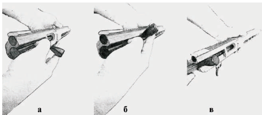
Рис. 138. Від'єднання затвора
