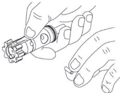
Рис. 39. Утримання викидача під час встановлення осі викидача
