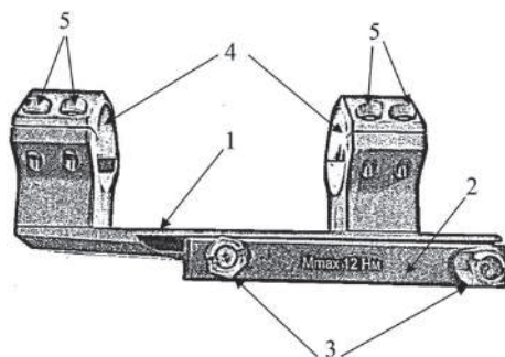
Рис. 47. Кронштейн для кріплення оптичного прицілу: 1 – корпус кронштейна; 2 – планка фіксуєча; 3 – гайки; 4 – кільця; 5 – гвинти фіксації оптичного прицілу
