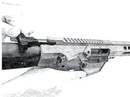
Рис. 12. Відведення важеля перезаряджання. Перевірка патронника
