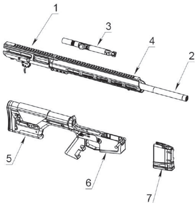
Рис. 133. Основні частини:
