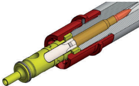
Рис. 32. Патрон в патроннику, затвор закритий
