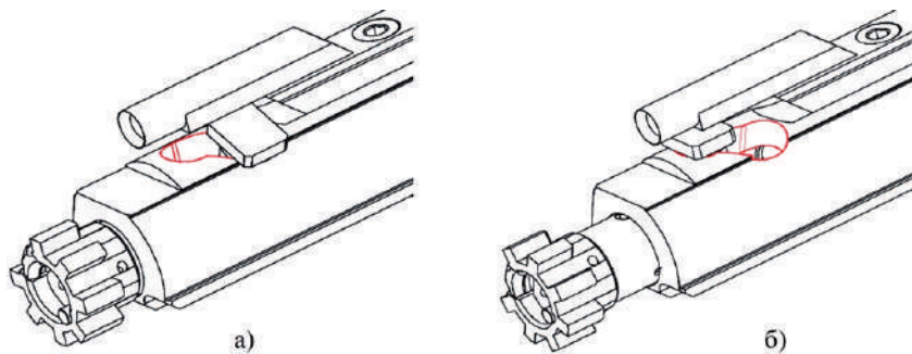
Рис. 101. Копірний паз в затворній рамі:
