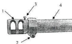
Рис. 155. Дульне гальмо – компенсатор:
