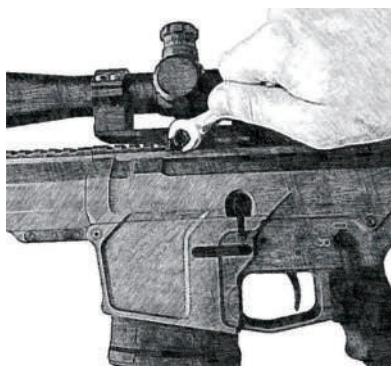
Рис. 48. Встановлення кронштейна на гвинтівку
