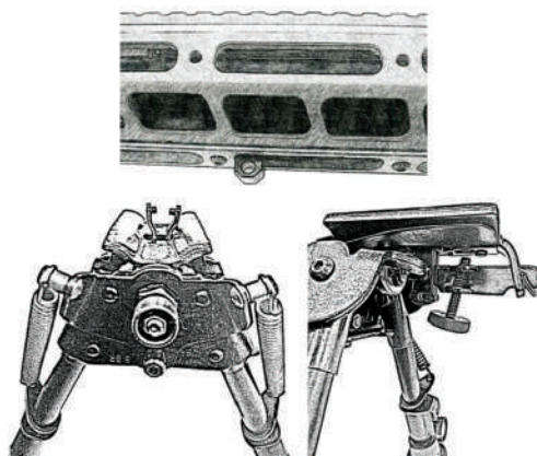
Рис. 159. Вузол кріплення сошок до антабки гвинтівки
