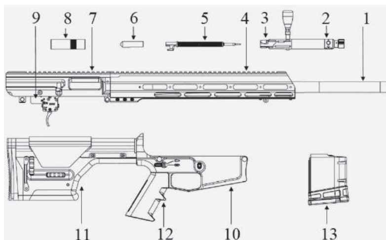
Рис. 142. Гвинтівка у розібраному стані (неповне розбирання):
