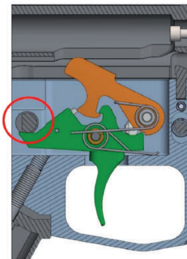
Рис. 35. Постановка гвинтівки на запобіжник, рух спускового гачка заблоковано, курок на бойовому зводі
