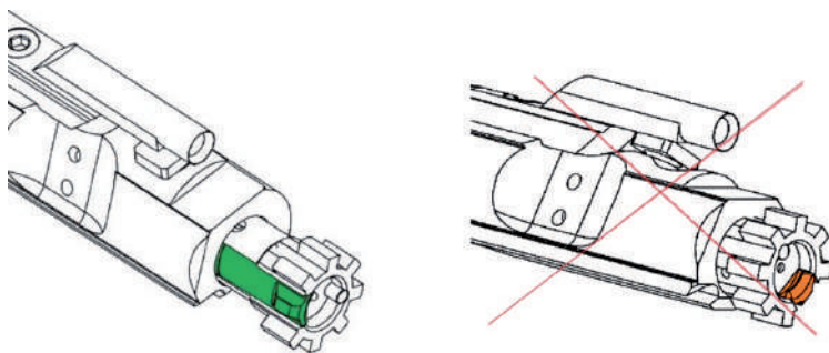
Рис. 91. Положення затвору при збиранні із затворною рамою
