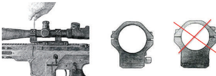
Рис. 49. Фіксація оптичного прицілу в кронштейні Зазор зліва і справа на одному кільці має бути однаковий і становить приблизно 1,6 мм
