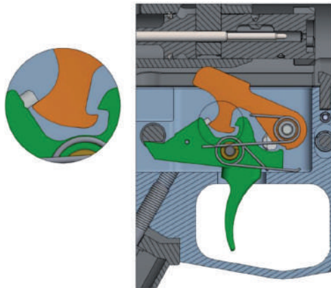
Рис. 30. Зачеплення курка та шпателя одиночного вогню (спусковий гачок натиснутий)
