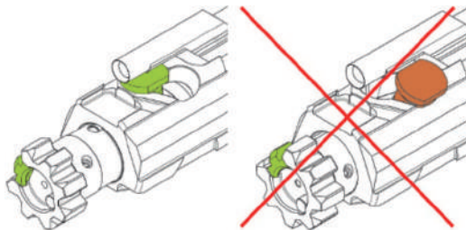
Рис. 25. Положення деталей затворної рами під час збирання з рамою верхньою
