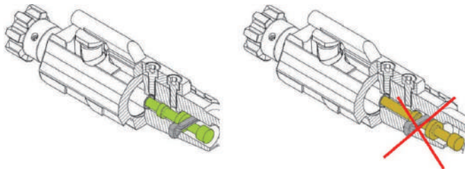
Рис. 24. Фіксація ударника штифтом при збиранні затворної рами
