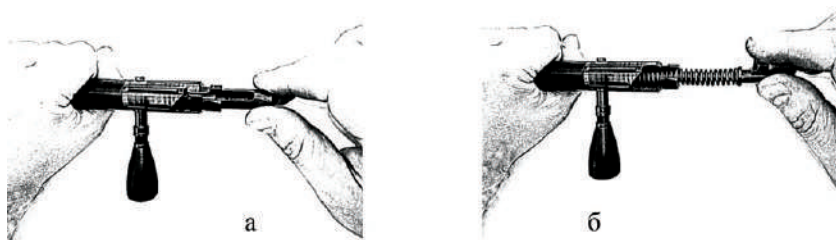
Рис. 140. Від'єднання упора пружини бойової та ударника в зібраному стані
