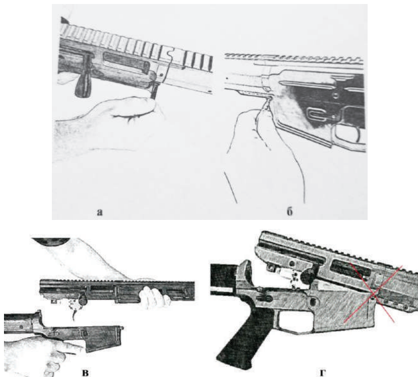
Рис. 137. Розділення ствольної коробки на нижню та верхню рами
