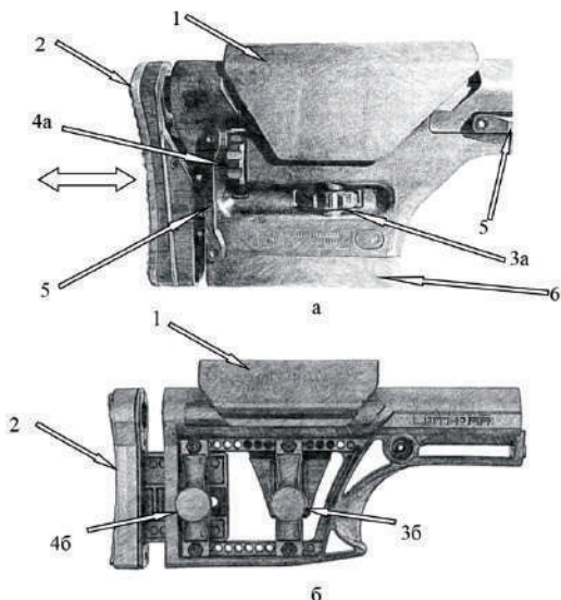
Рис. 50. Приклад UAR-10 та його основні частини:
