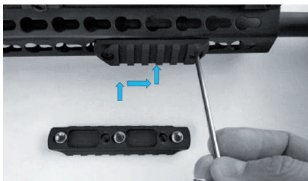
Рис. 59. Кріплення планки «пікатіні» на цівку з кріпленням типу кеймод (KeyMod)
