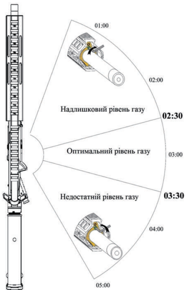
Рис. 124. Схема напрямку викидання гільзи
