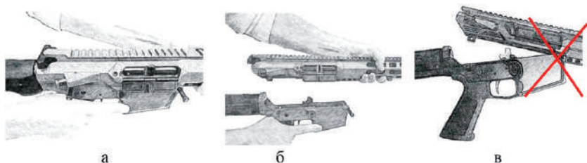
Рис. 13. Роз'єднання ствольної коробки
