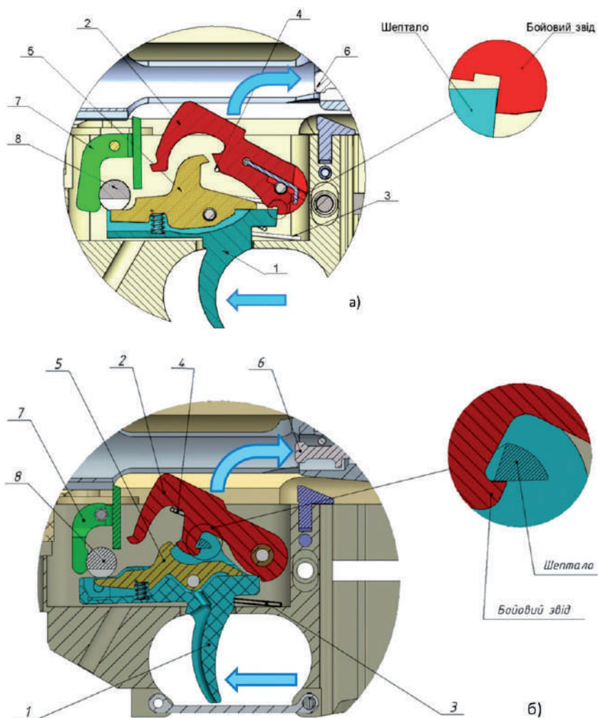
Рис. 96. Дія спускових механізмів (деталі в положенні – готовий до пострілу):
