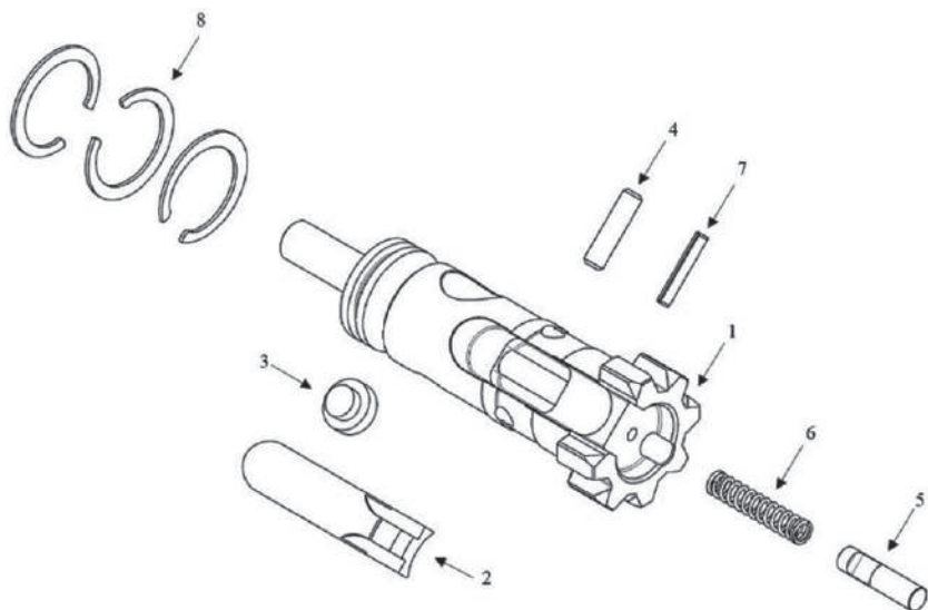
Рис. 36. Затвор у розібраному стані:
