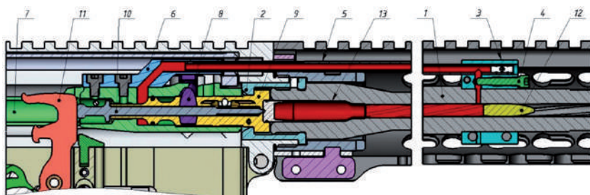
Рис. 74. Будова автоматики гвинтівки UAR-15 (зображене на схемі положення: затвор зчеплений з муфтою бойових упорів)
