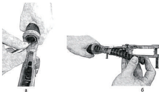
Рис. 19. Від'єднання буфера віддачі і зворотної пружини
