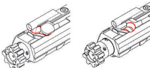
Рис. 29. Копірний паз в затворній рамі
