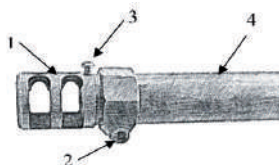
Рис. 40. Дульне гальмо-компенсатор:
