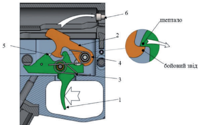
Рис. 28. Дія спускового механізму (деталі УСМ в положенні до пострілу):
