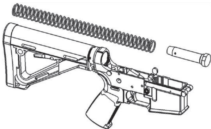
Рис. 88. Рама нижня, буфер віддачі та зворотна пружина роз'єднані
