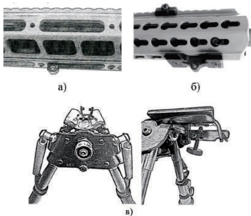
Рис. 45. Кріплення сошок до антабки гвинтівки: а) антабка UAR-10; б) антабка UAR-10М; в) вузол кріплення сошок
