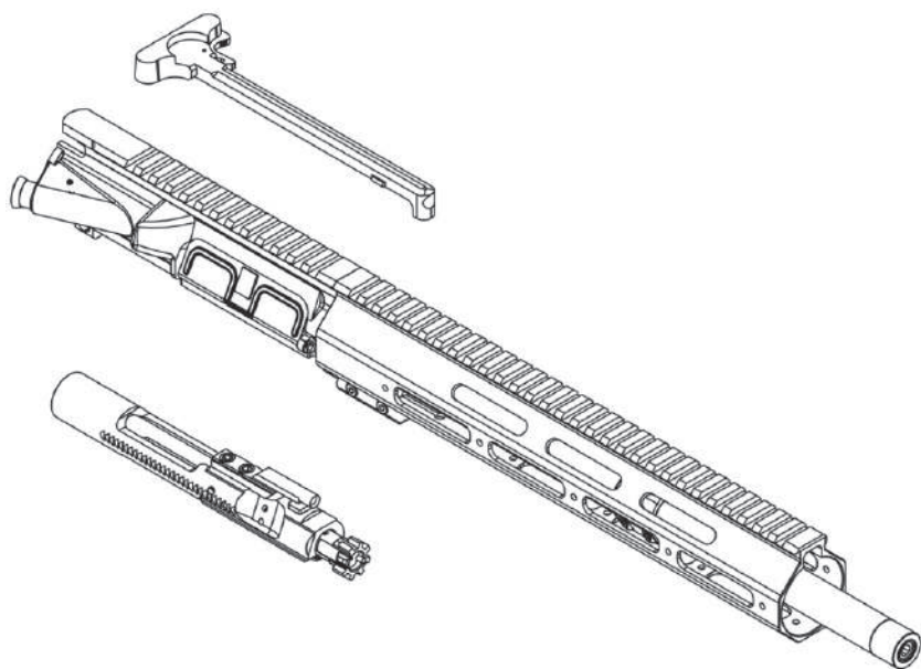
Рис. 82. Верхня рама ствольної коробки, затворна рама із затвором у зборі та важіль перезарядження
