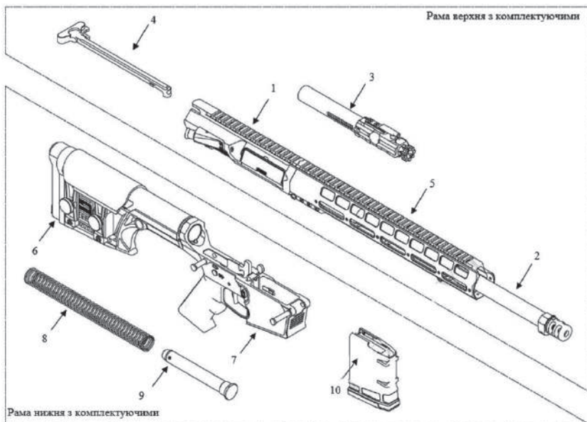
Рис. 8. Основні частини:
