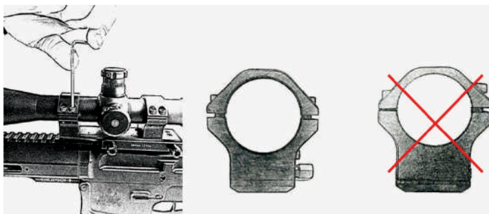
Рис. 163. Фіксація оптичного прицілу в кронштейні. Зазор зліва і справа на одному кільці має бути однаковий і становить приблизно 1,6 мм
