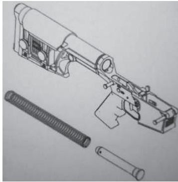
Рис. 20. Нижня частина рами, буфер віддачі та зворотна пружина від'єднанні.
