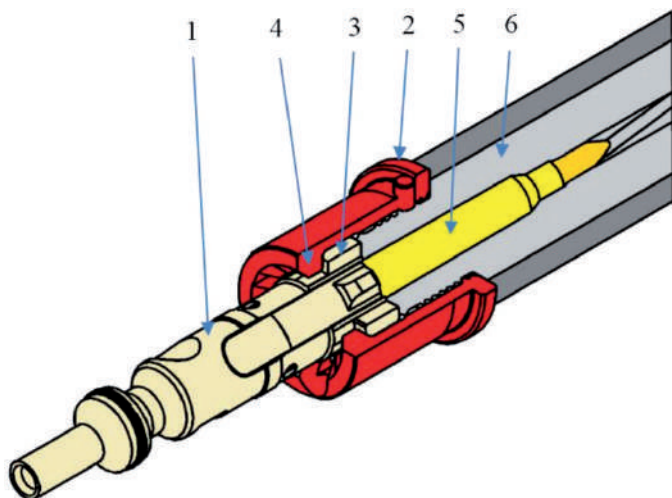
Рис. 103. Патрон в патроннику, затвор закритий:
