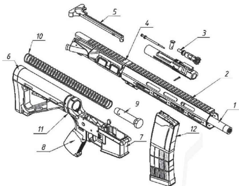
Рис. 89. Автоматична гвинтівка – неповне розбирання:
