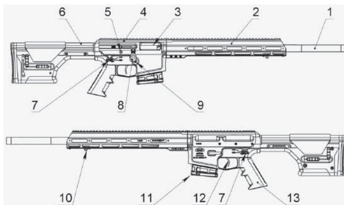
Рис. 132. Органи керування та елементи будови гвинтівки UBR-008:
