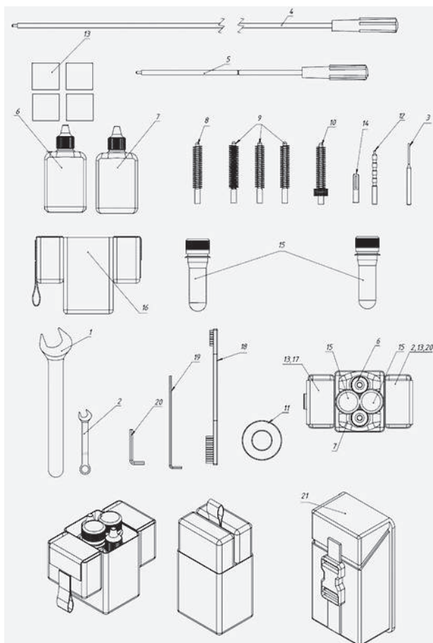
Рис. 174. Комплект засобів для чищення
