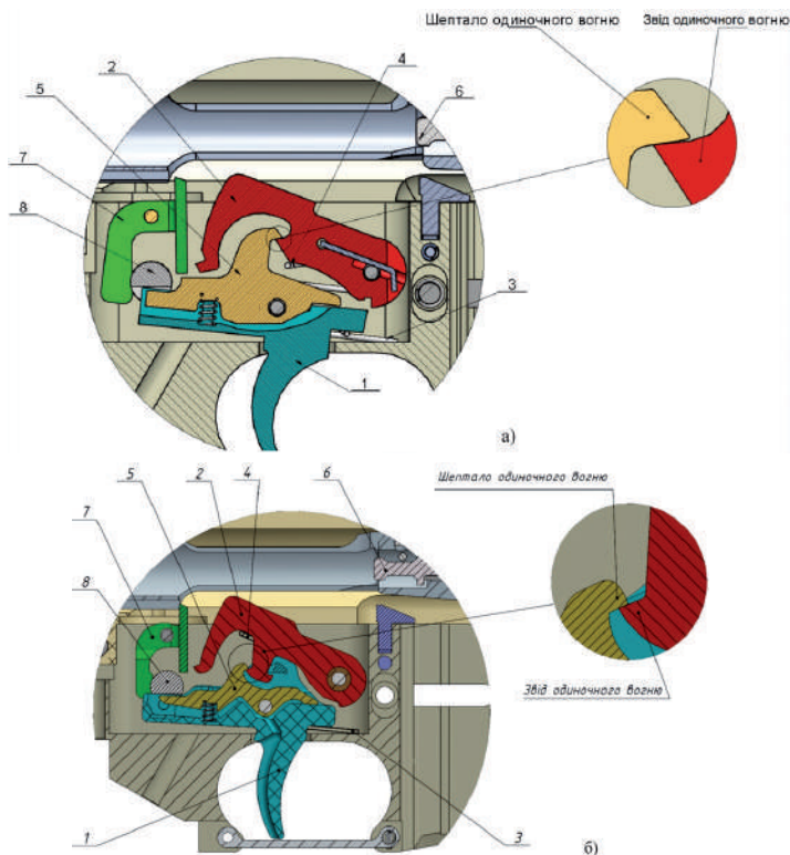
Рис. 102. Зачеплення курка та шептала одиночного вогню (спусковий гачок натиснутий):
