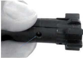
Рис. 109. Утримання викидача при знятті осі викидача
